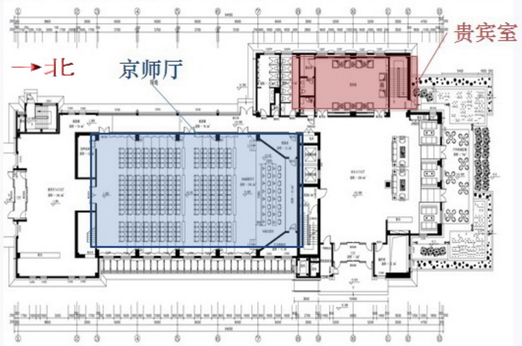
京师学堂一层平面图
